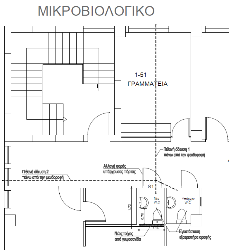
Σκαρίφημα. 2: Πιθανές οριζόντιες οδεύσεις σωληνώσεων εξαεριστήρων W.C.
