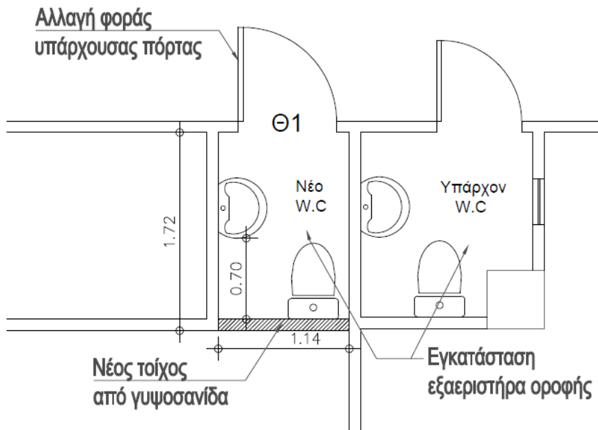
Σκαρίφημα. 1: Διαμόρφωση νέου χώρου W.C.
